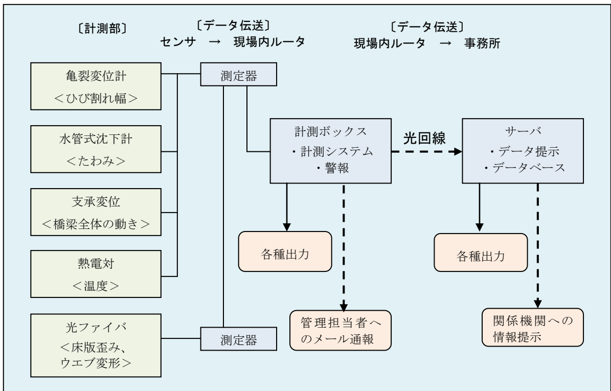
図 4-13 システム構成図
