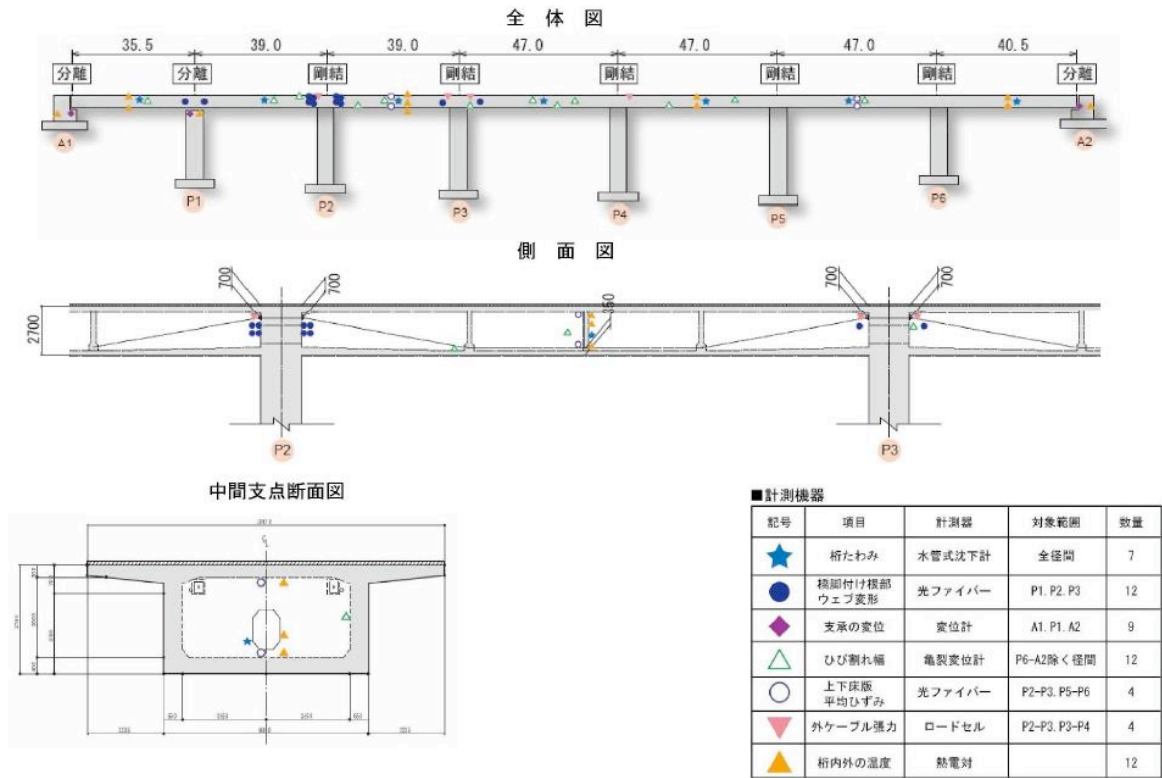
図 4-12 計器の配置図
